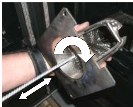
Fig. 115 : nettoyage du pot brûleur
