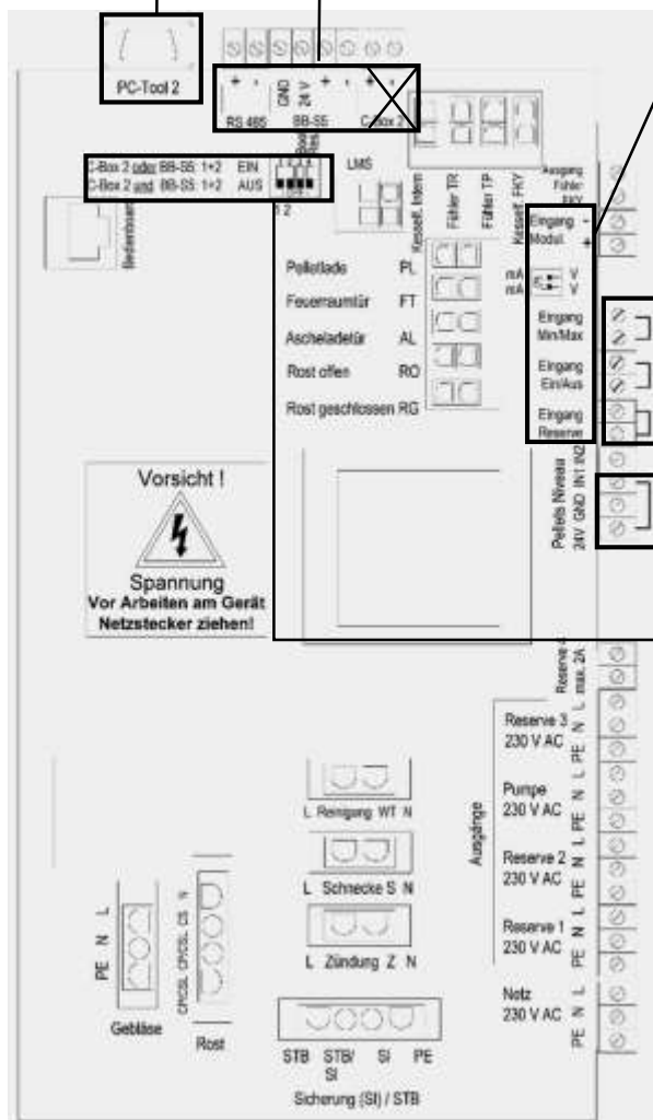
Fig. 50 : entrées carte-mère
