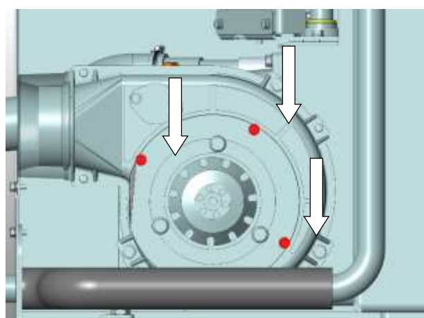
Fig. 145 : vissages soufflerie
