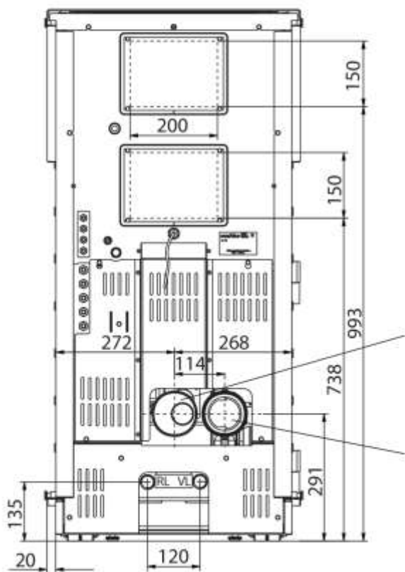
Fig. 150 : plan coté ivo.tec®
