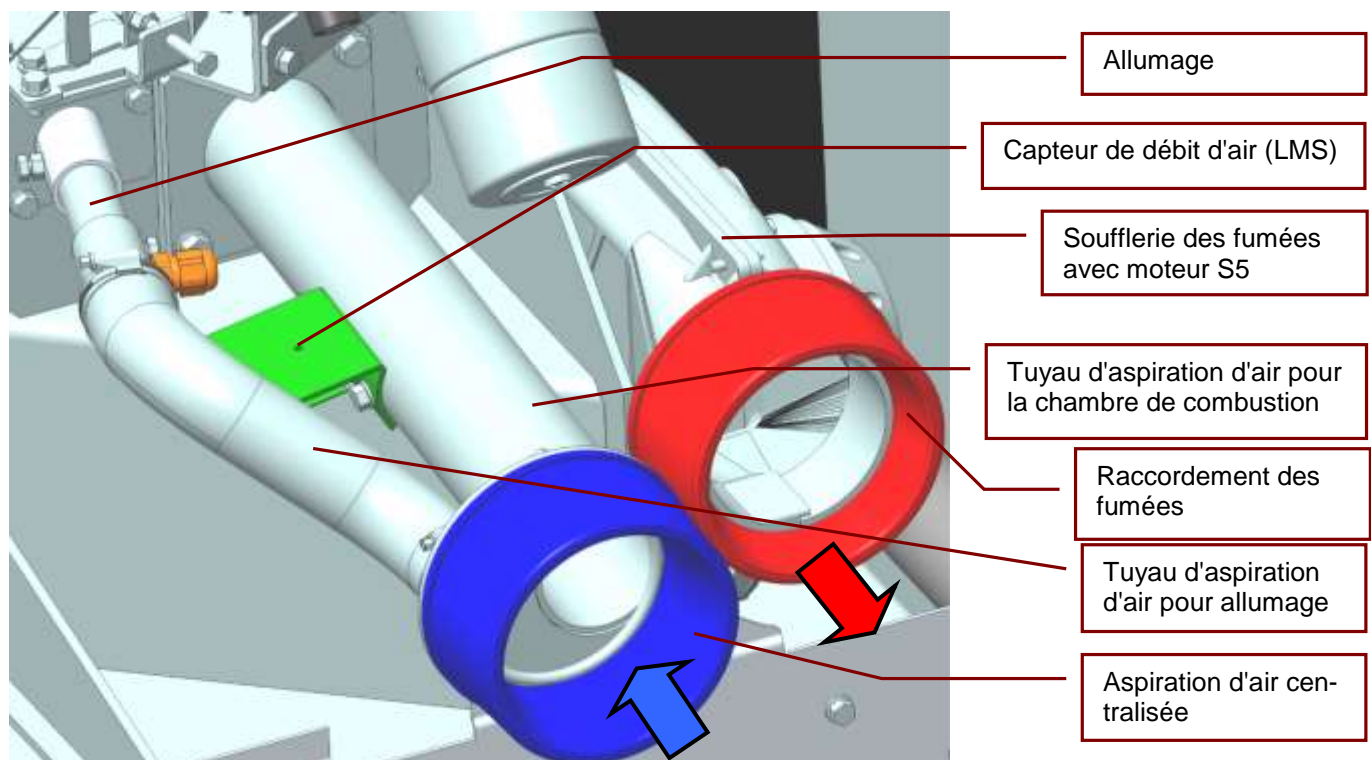
Fig. 143 : manchon d'admission d'air et d'air vicié BM 01
