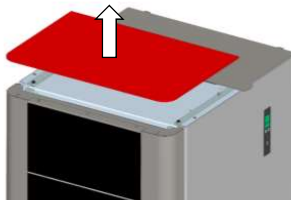
Fig. 19 : démontage du couvercle
