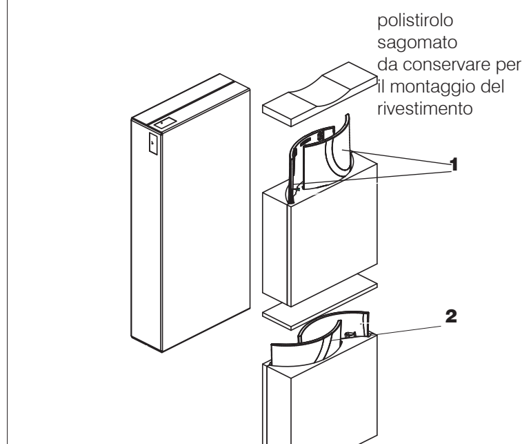
scatola coi fianchi in ceramica
