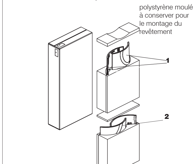
boîte avec les flancs en céramique
