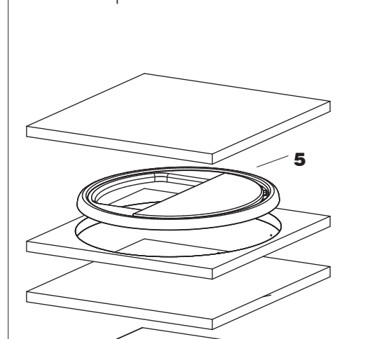
scatola col top in ceramica
