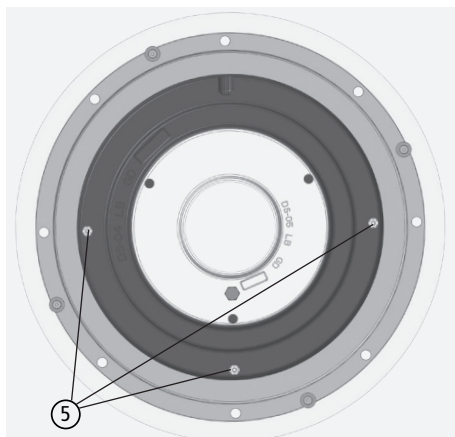
Fig. 3.8 Goujons filetés dans la partie haute du socle pivotant (vue de dessus)
