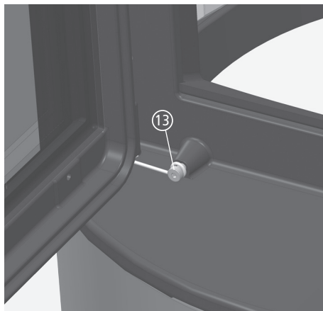
Fig. 3.29 ressort de porte sous tension
