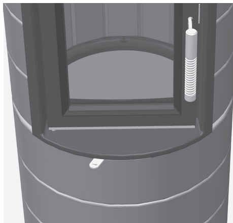
Fig. 4.3 Registre d'air de combustion : à gauche = complètement fermé
