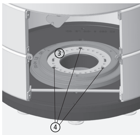
Fig. 3.17 Retirer la rondelle de réglage des butées latérales
