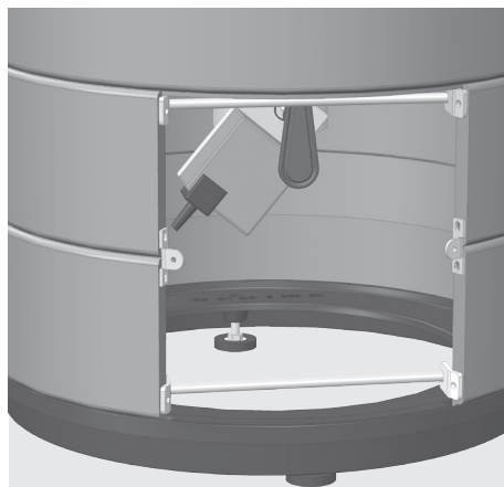
Fig. 3.2 Pieds de réglage sous la sole de l'appareil, plaque de couverture enlevée
