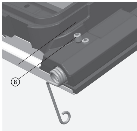
Fig. 3.26 Sécuriser le ressort de porte
