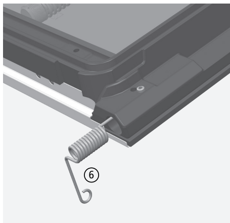
Fig. 3.25 Insérer le ressort de porte
