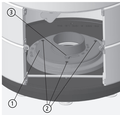
Fig. 3.12 socle pivotant, partie haute
