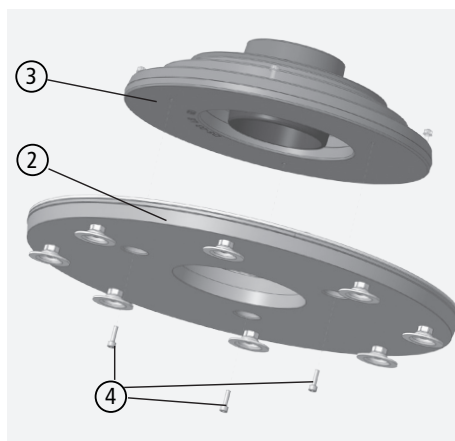
Fig. 3.6 Socle pivotant avec console de base et partie supérieure
