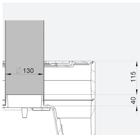
Fig. 3.46 Distance entre l'ajutage des gaz brûlés et la plaque de couverture
