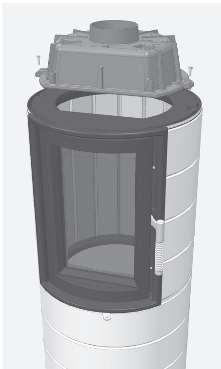
Fig. 3.31 Montage du dôme en fonte (échangeur de chaleur)
