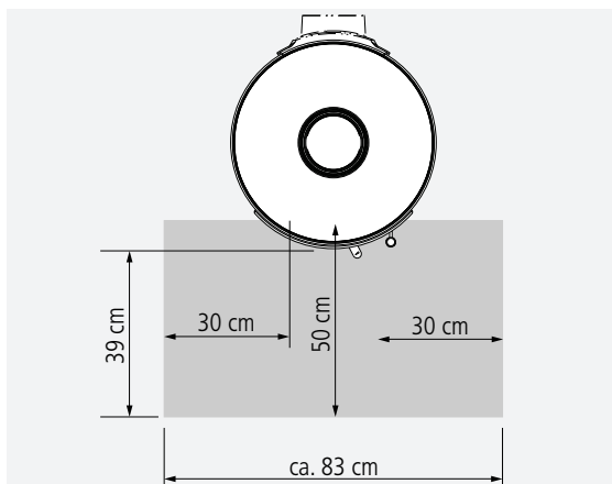
Fig. 1.2 Revêtement non inflammable devant et à côté de l'ouverture de foyer
