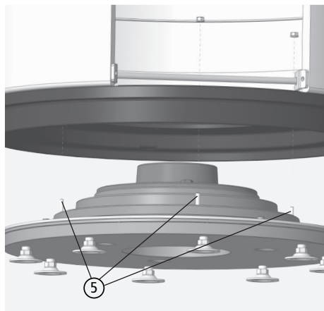
Fig. 3.7 Goujons filetés dans la partie haute du socle
