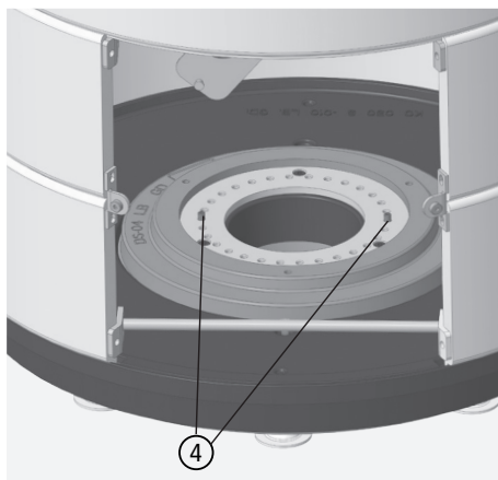
Fig. 3.13 Vis de butée, réglage des butées gauche et droites
