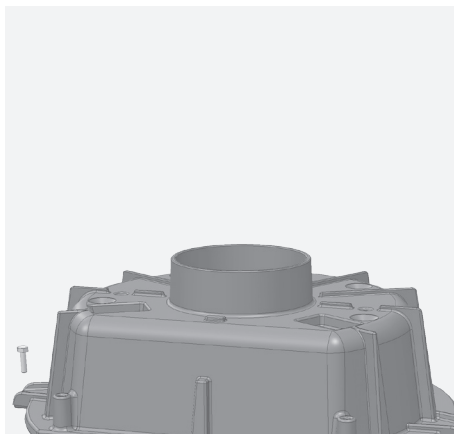
Fig. 3.3 Buse pivotante de sortie des fumées pivotante à monter sur le dôme en fonte (échangeur à chaleur)
