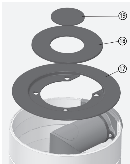
Fig. 3.44 Plaque de couverture en fonte
