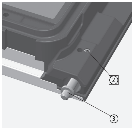
Fig. 3.23 Enlever la tige de charnière inférieure
