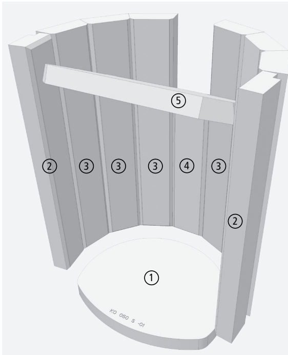
Fig. 5.2 Garnissage de foyer et déflecteur
