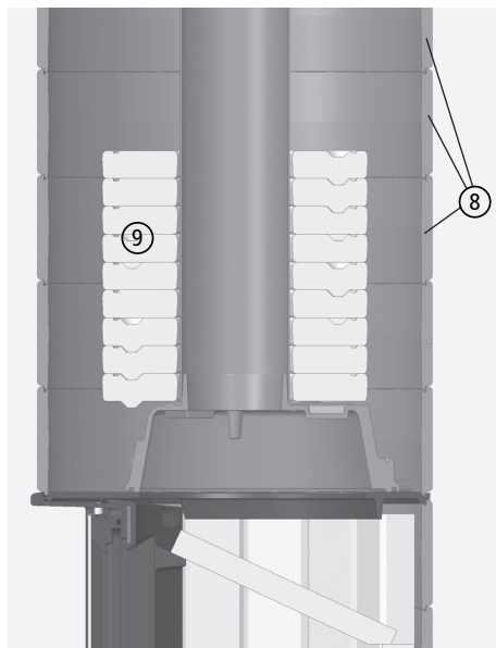
Fig. 3.39 Rehausse avec 6 anneaux en fonte et 9 pièces intercalaires d'accumulateur
