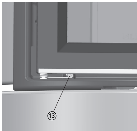
Fig. 3.28 Mise sous tension du ressort de porte
