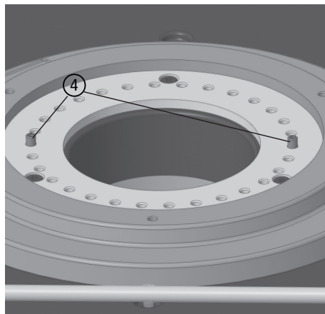
Fig. 3.14 Goupilles d'arrêt, réglage des butées d'extrémité gauche et droite
