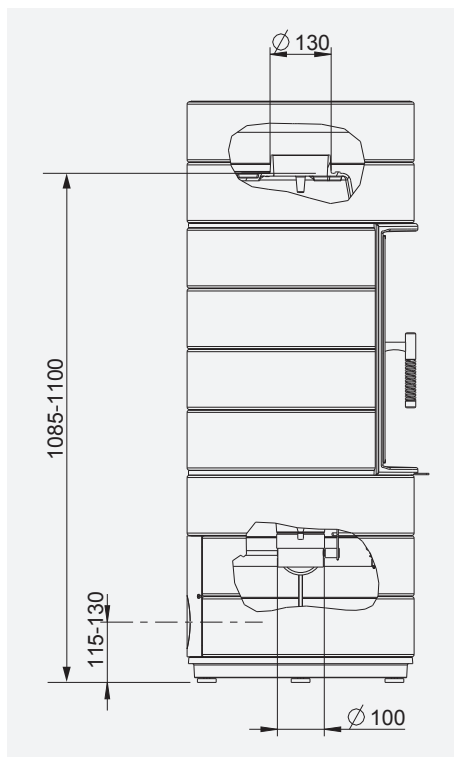
Fig. 3.45 Raccord de gaz brûlés pour le COLONA lite avec 2 anneaux en fonte
