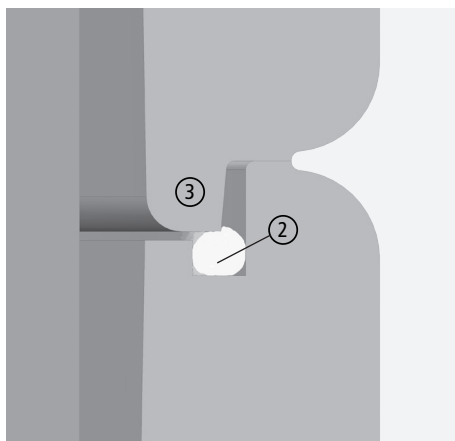
Fig. 3.36 Encoche/gorge dans l'anneau en fonte, rebord de l'anneau en fonte posé dessus
