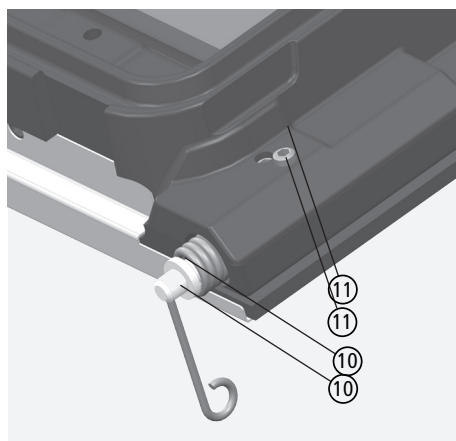
Fig. 3.27 Tige charnière et ressort de porte
