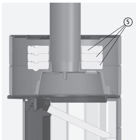
Fig. 3.37 Rehausse avec 2 anneaux en fonte et 3 pièces intercalaires d'accumulateur
