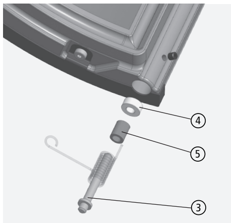
Fig. 3.24 Tige de charnière inférieure avec les douilles entretoise
