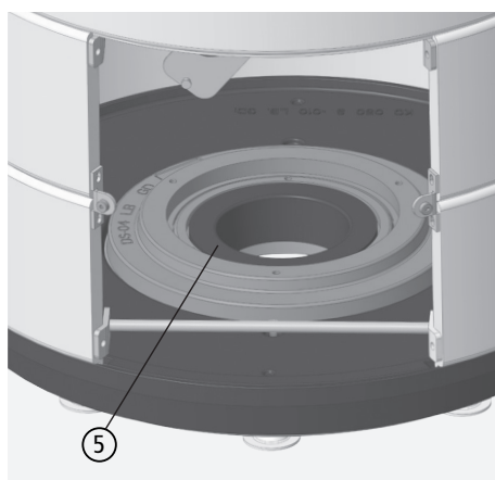
Fig. 3.18 Raccord d'air de combustion, vers le bas
