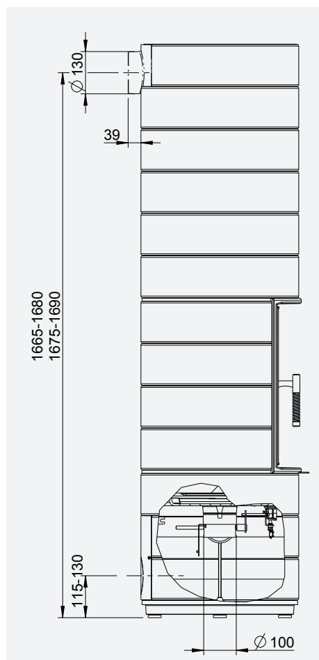
Fig. 3.47 Raccord de gaz brûlés pour le COLONA lite avec 6 anneaux en fonte
