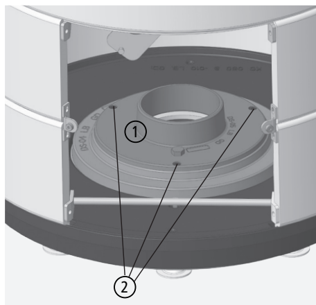
Fig. 3.16 Retirez la partie supérieure du support pivotant
