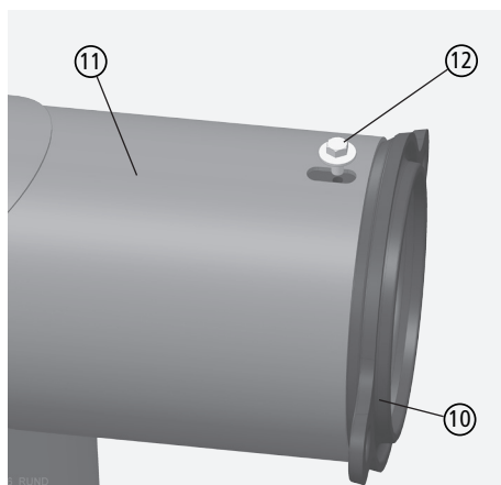
Fig. 3.41 Fixation du tuyau des gaz de chauffage sur la tubulure de raccordement en fonte
