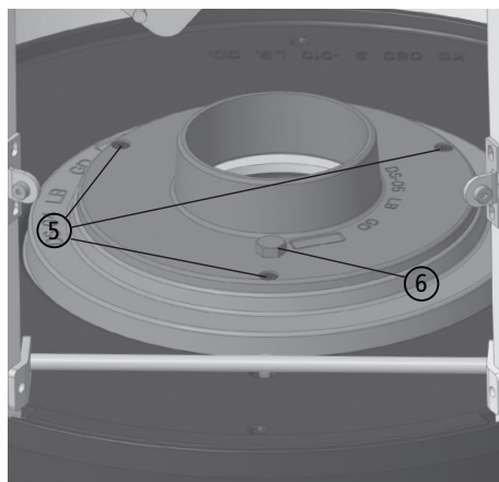
Fig. 3.15 Monter la partie haute du socle pivotant
