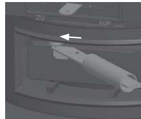
Fig. 4.15 Grille à secousses : levier à gauche = grille fermée
