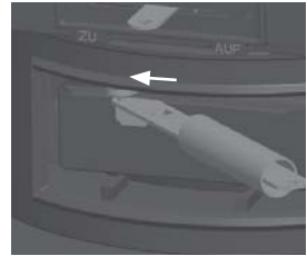
Fig. 4.21 Grille à secousses : levier à gauche = grille fermée
