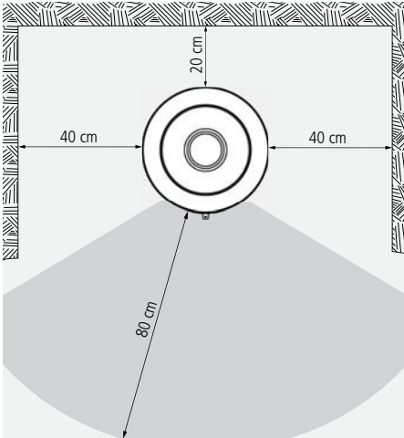
Fig. 1.3 Mindestabstände im Bereich der Sichtscheibe
