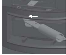
Fig. 4.13 Grille à secousses : levier à gauche = grille fermée
