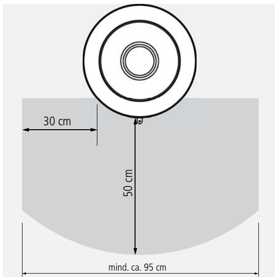
Fig. 1.2 Revêtement non inflammable devant l'ouverture du foyer
