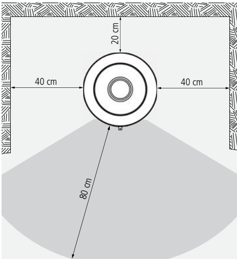
Fig. 1.1 Distances minimales par rapport aux matériaux ou composants inflammables
