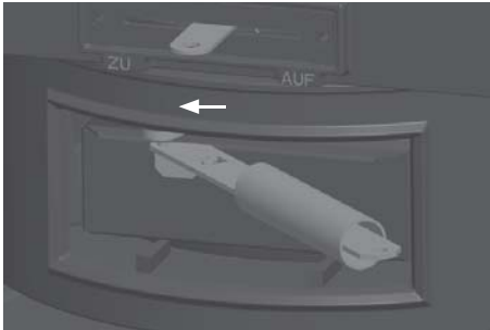
Fig. 4.4 Grille à secousses fermée pour le fonctionnement au bois de chauffage.
