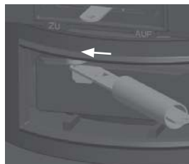
Fig. 4.11 Grille à secousses : levier à gauche = grille fermée
