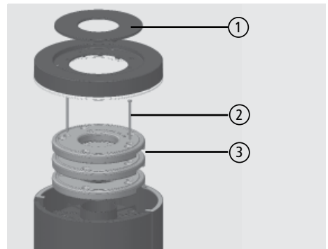
Fig. 3.1 Démontage de recouvrement
