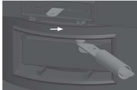
Fig. 4.5 Grille à secousses ouverte pour le fonctionnement à la lignite
