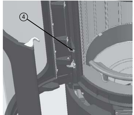
Fig. 3.5 Vis du ressort de porte
