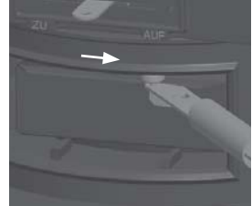
Fig. 4.17 Grille à secousses : levier à droite = grille et air inférieur ouverts
