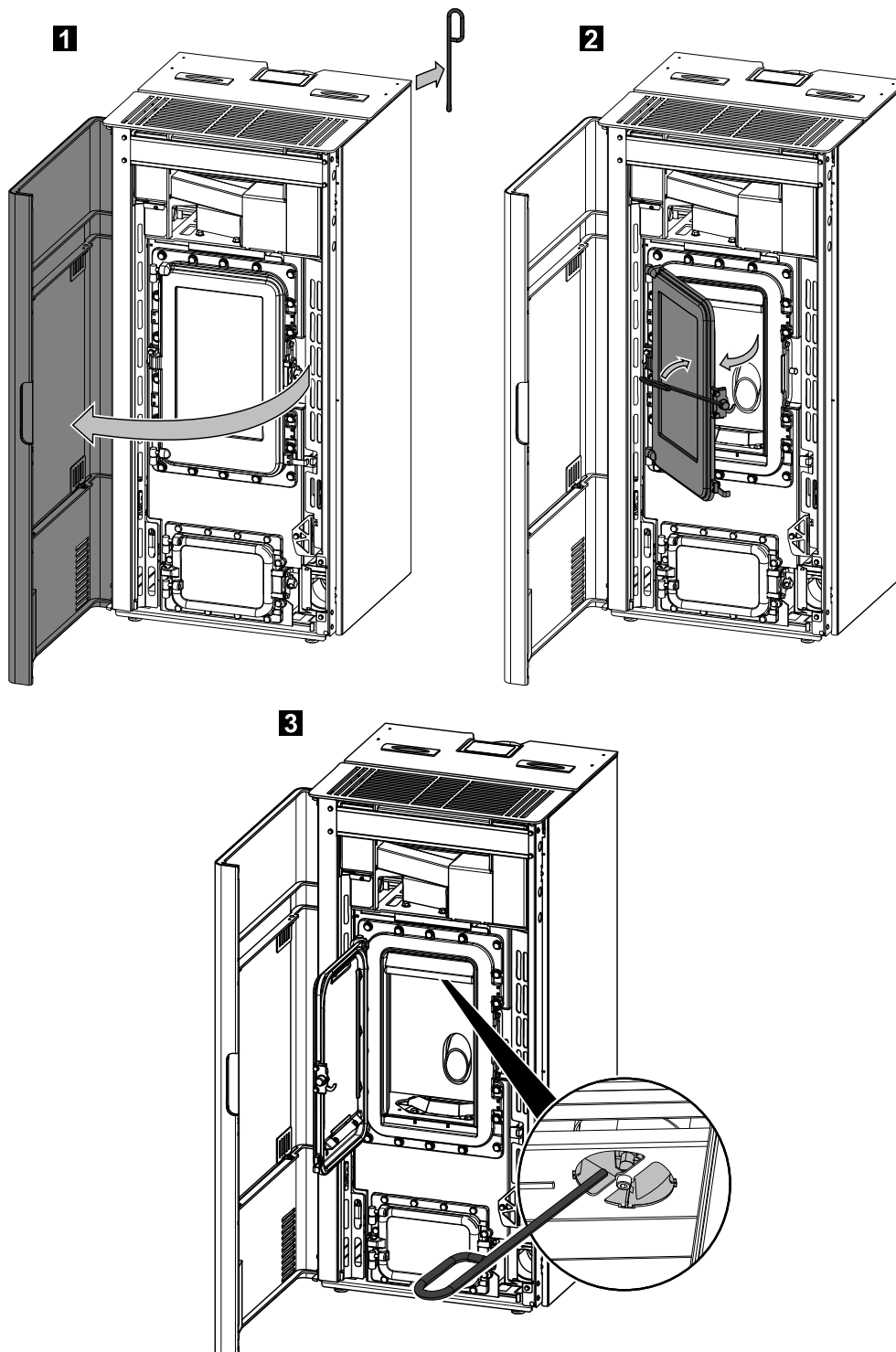
Illustration 4: Nettoyage de la plaque déflectrice
