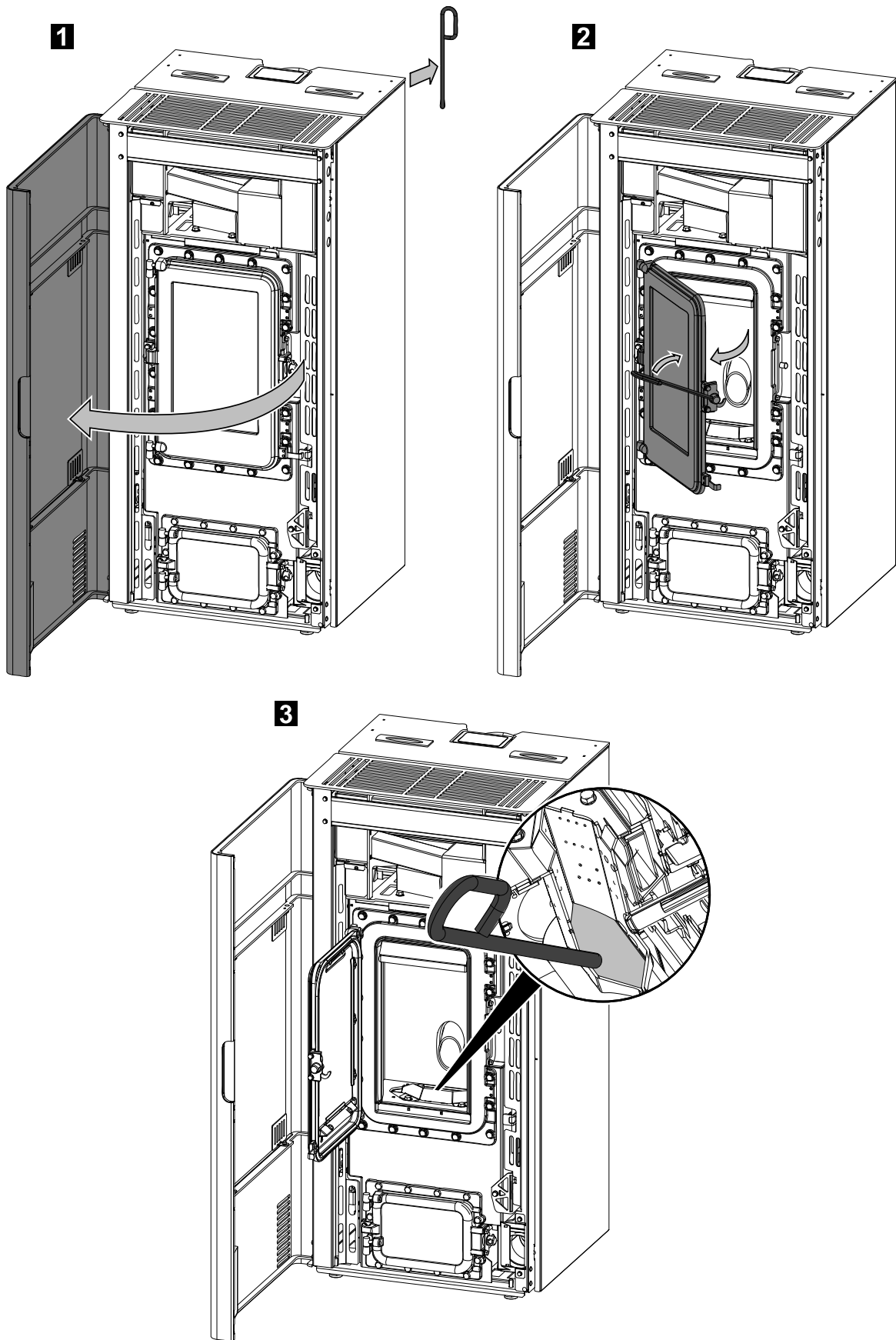
Illustration 1: Nettoyage du brûleur (à l'aide de l'outil fourni)
