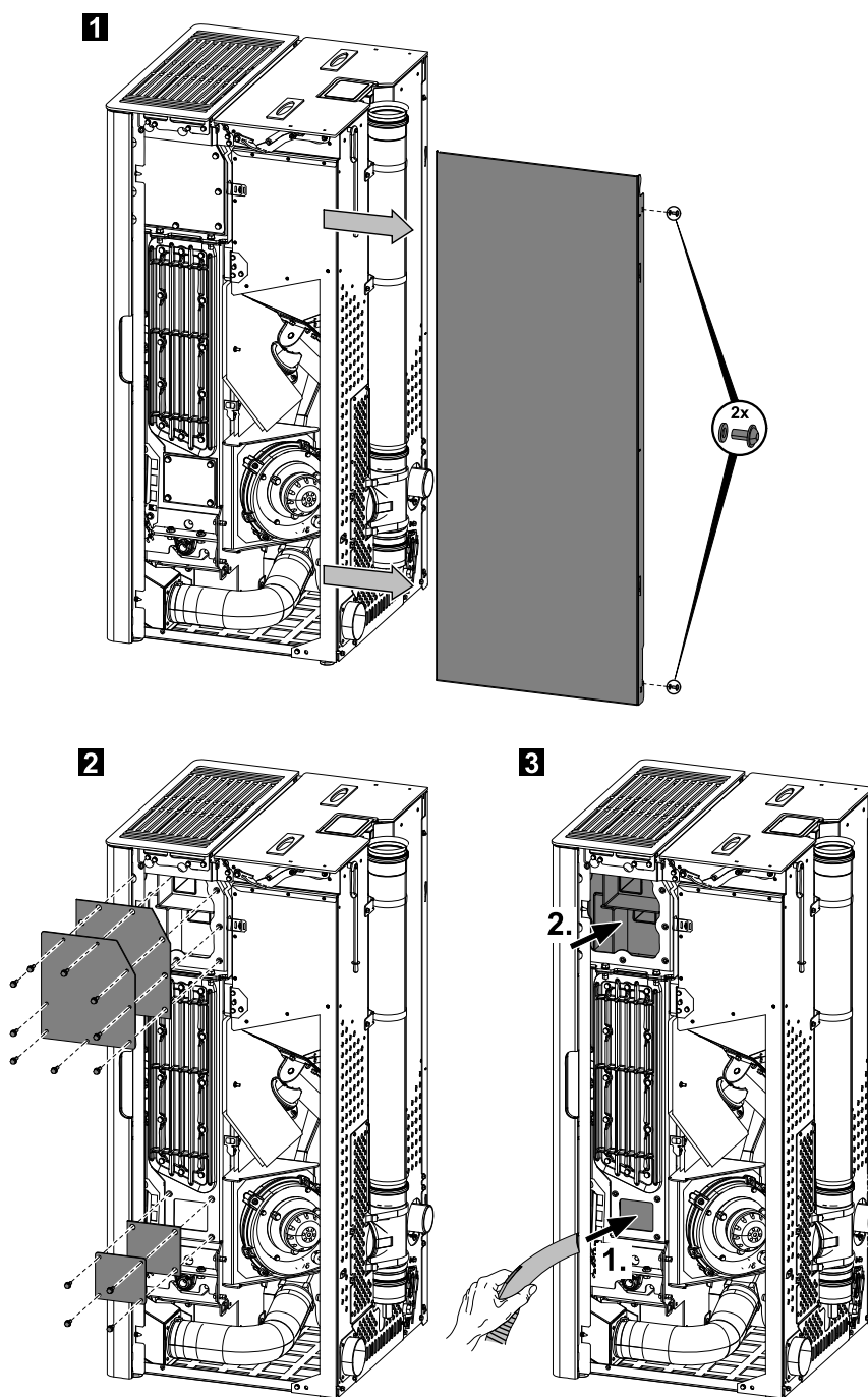
Illustration 3: Démontage de la paroi extérieure arrière
