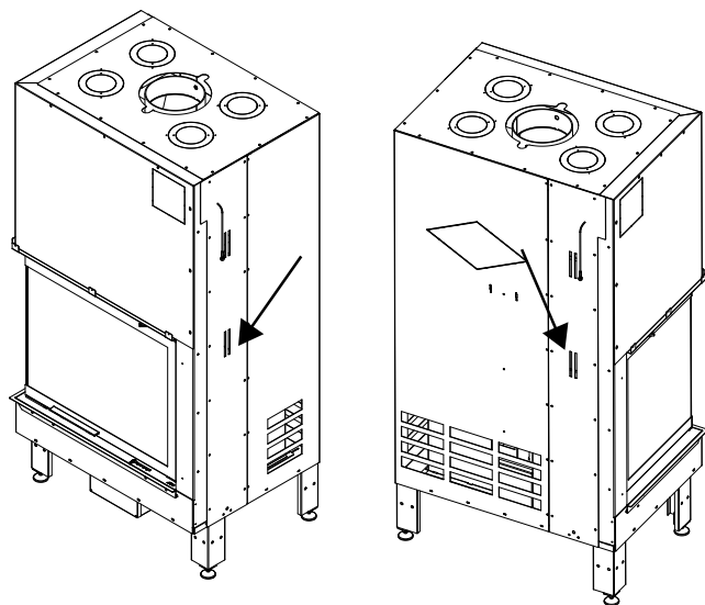
VIS DE BLOCAGE DES CONTREPOIDS
