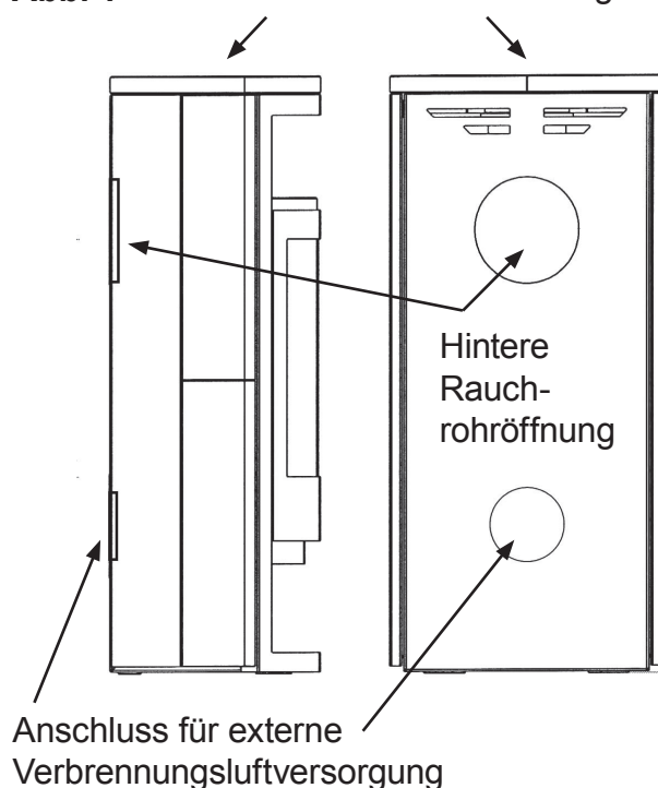
Abb. 1 Obere Rauchrohröffnung
