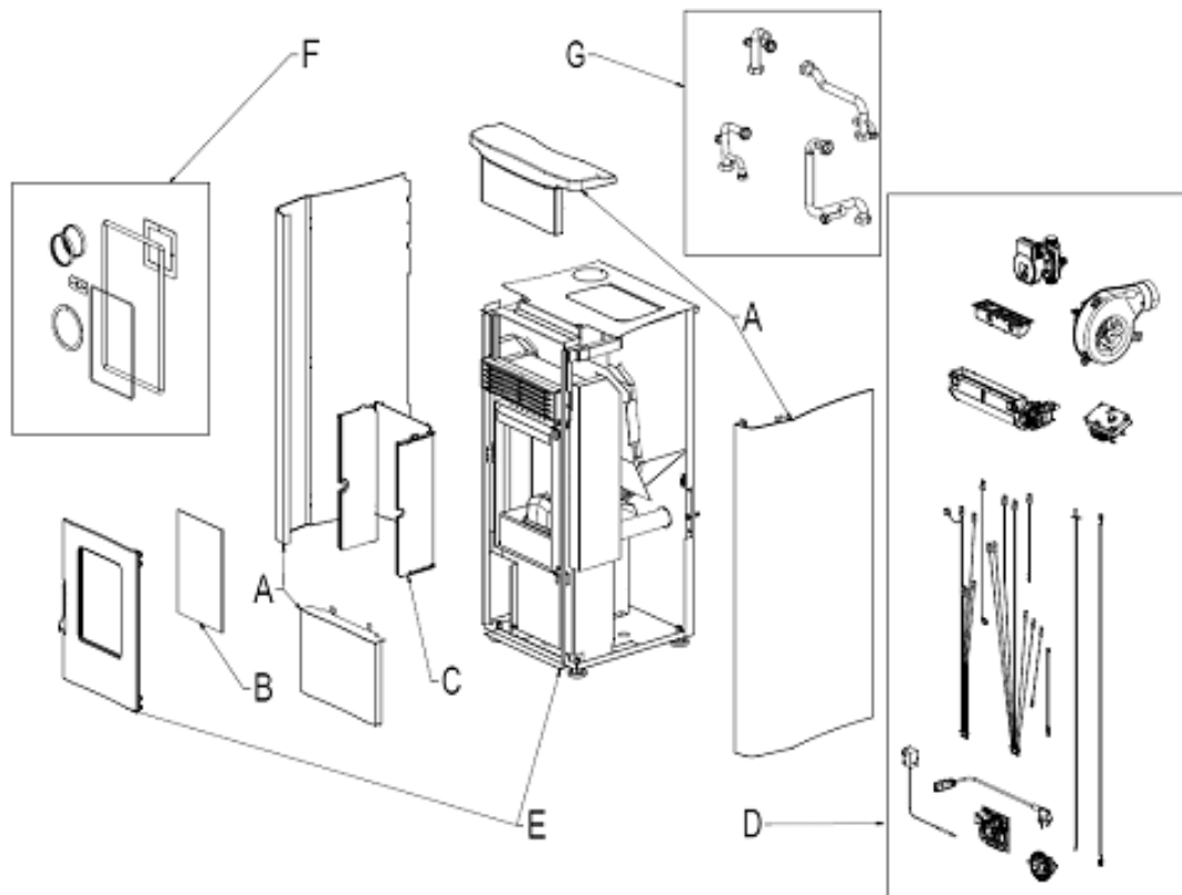
Fig. 1 - Dessin éclaté
