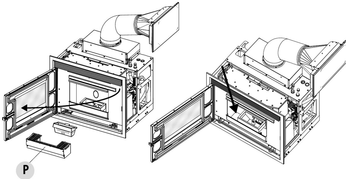
Fig. 19 - Tiroir à cendres
