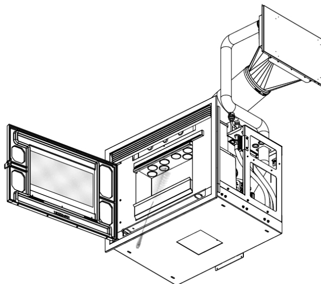
Fig. 22 - Nettoyage des faisceaux tubulaires
