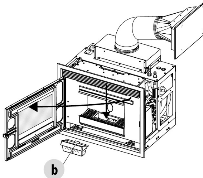
Fig. 18 - Nettoyage du brasier
