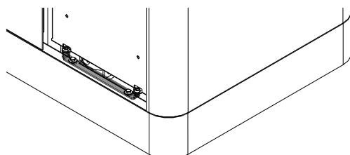
Fig. 105: Ajuster le support pour habillage en bas
