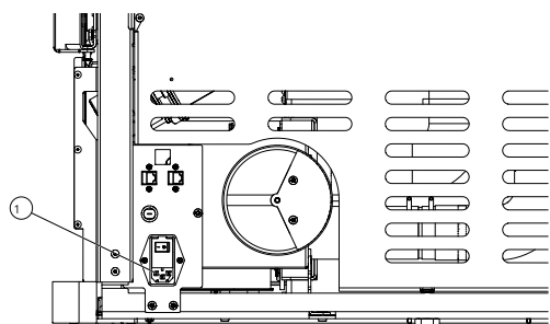
Fig. 50: Raccordement électrique
