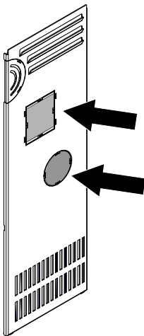
Fig. 40: Enlever les découpes perforées
