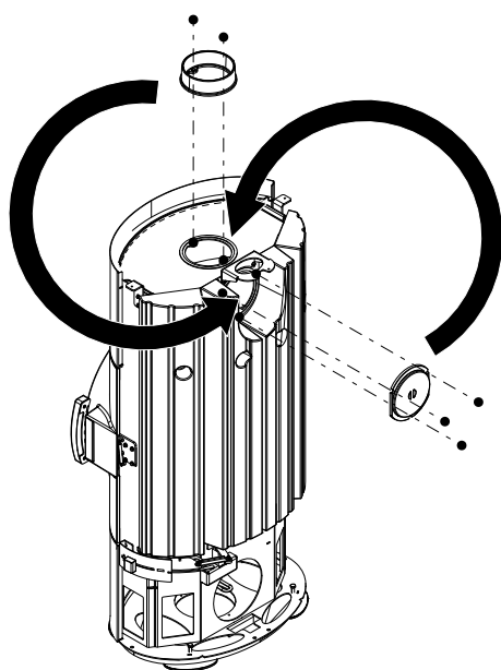
Fig. 12: Échanger le recouvrement et la tubulure
