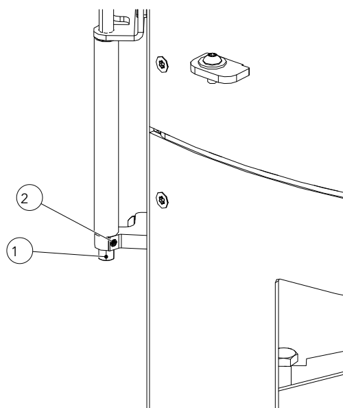
Fig. 27: Régler la force de fermeture de la porte
