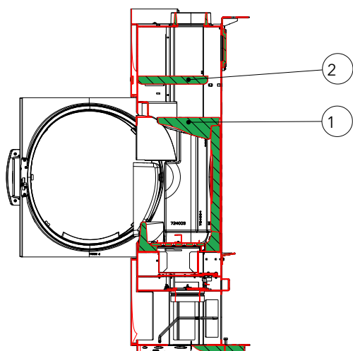
Fig. 39: Enlever la Keramott et la plaque déflectrice
