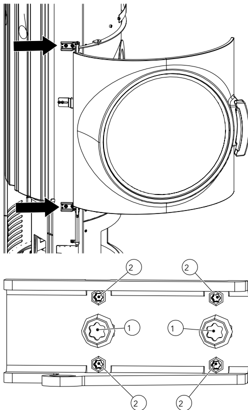
Fig. 22: Vis de réglage de la porte
