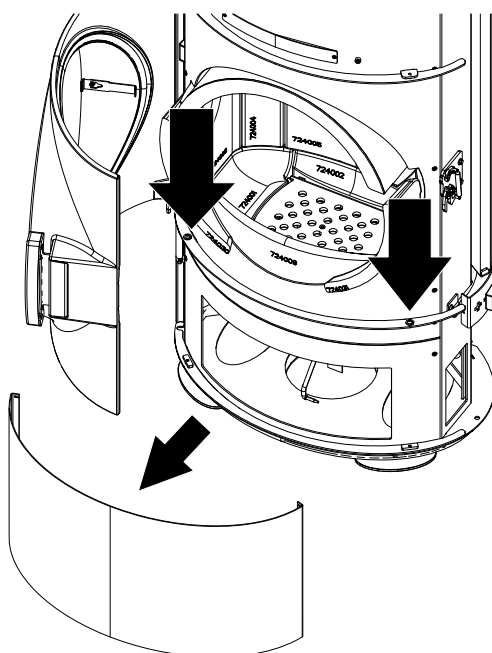
Fig. 21: Déposer l'habillage avant inférieur
