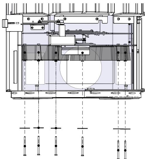
Fig. 7: Installer les pierres HMS en bas
