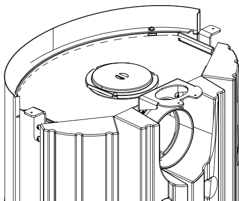
Fig. 13: Recouvrement et tubulure échangés
