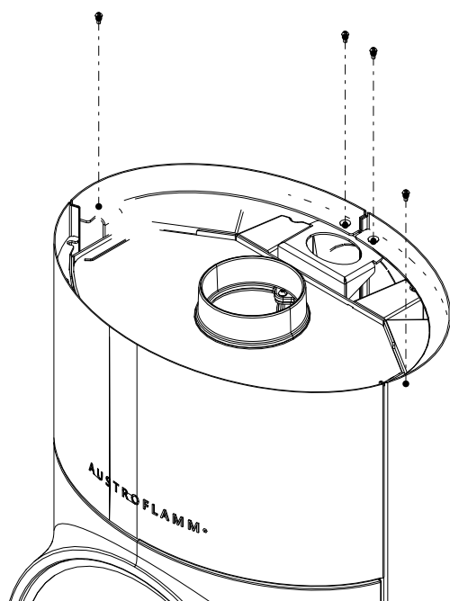
Fig. 37: Dévisser les vis
