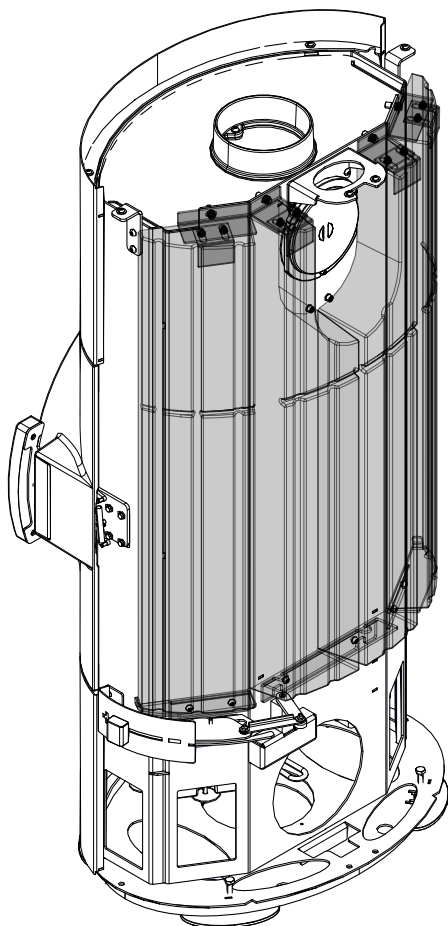
Fig. 6: Installer l'HMS
