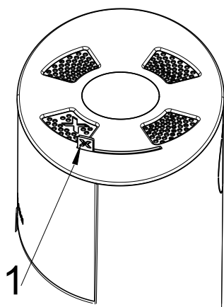
Fig. 35: Manette de régulation de l'air de convection
