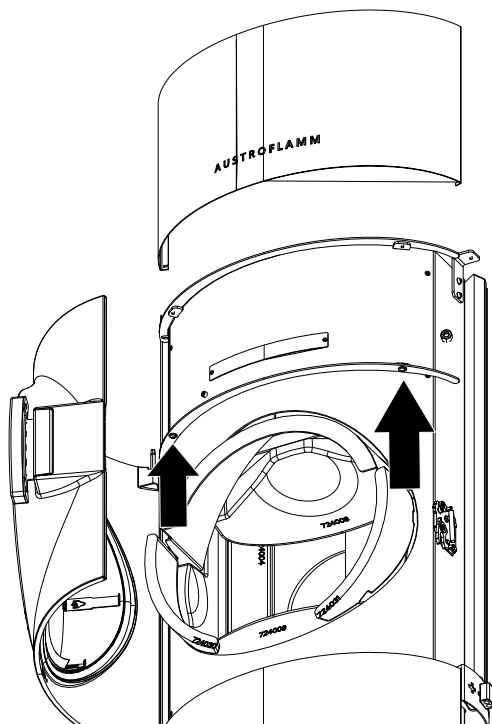
Fig. 20: Déposer l'habillage avant supérieur
