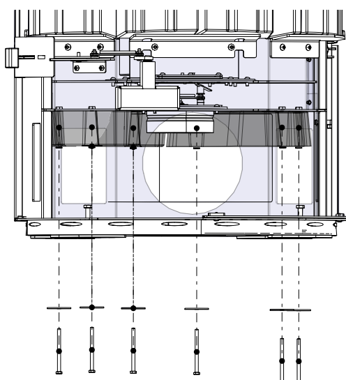
Fig. 42: Monter les pierres HMS en bas
