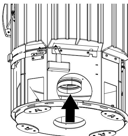
Fig. 16: Fixer le tuyau flexible en alu
