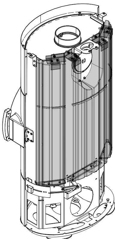
Fig. 41: Dévisser les vis et déposer l'HMS
