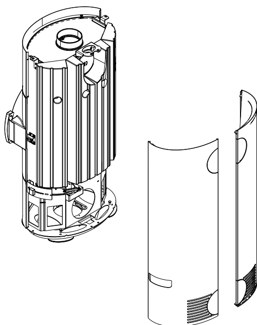
Fig. 38: Enlever l'habillage latéral
